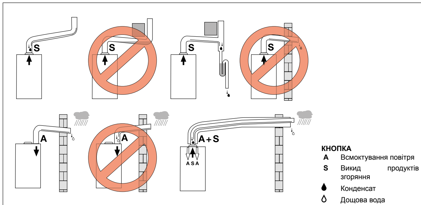
Рис. 13 Приклади монтажу
