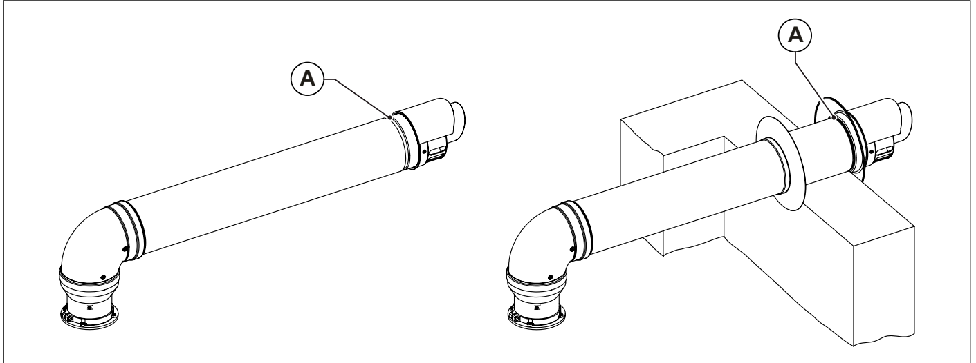
Рис. 15 Настінна установка терміналу
