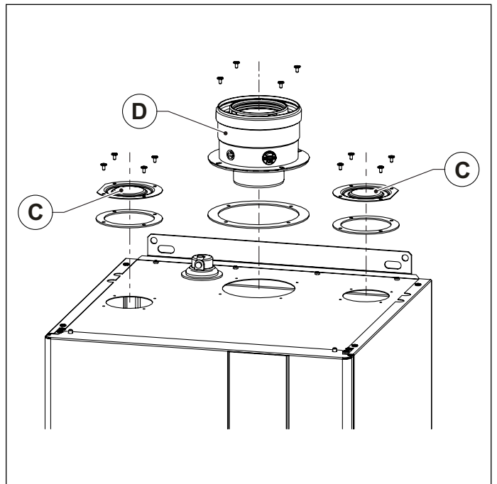
Рис. 12 Установка коаксіального набору
