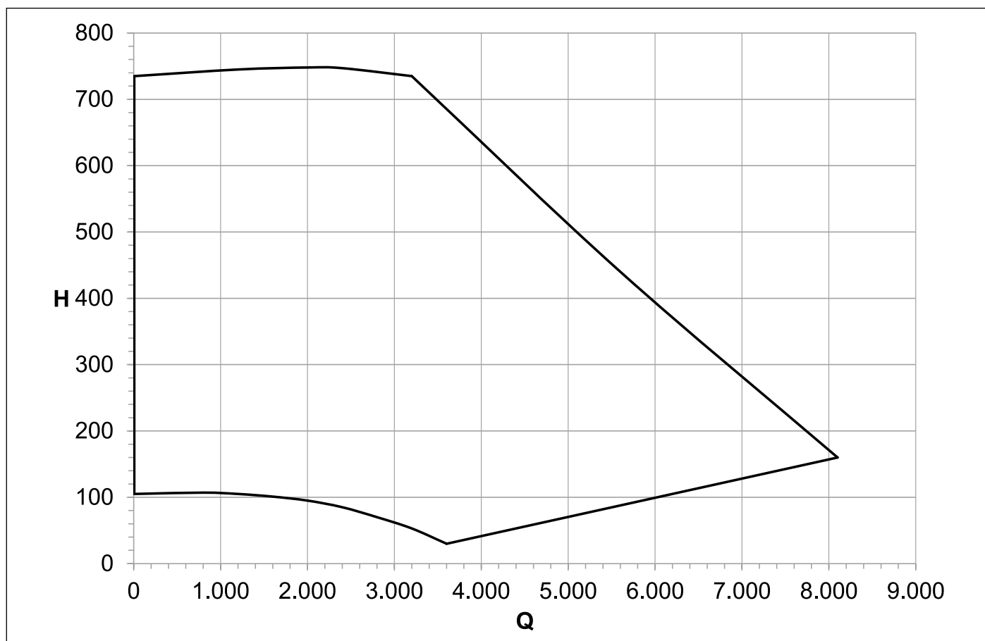
Рис. 24 Наявний напір YONOS PARA HF 25/7
