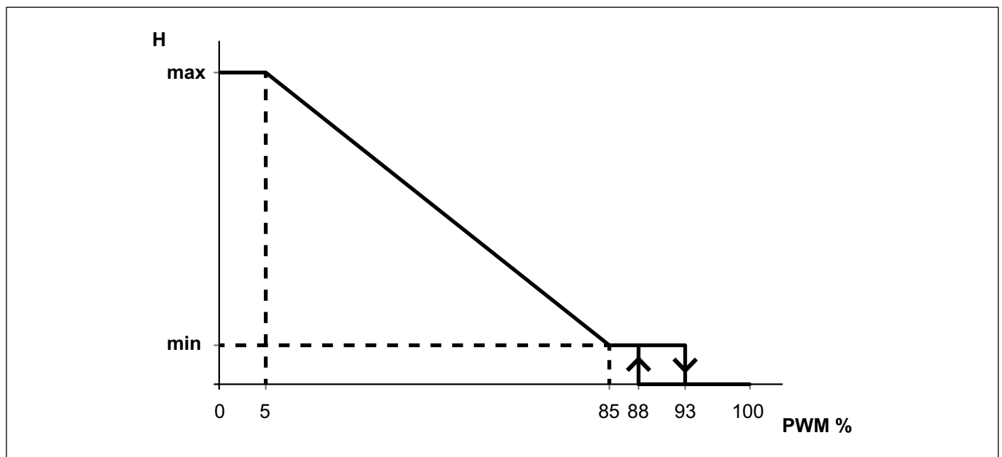
Рис. 25 Сигнал ШІМ
