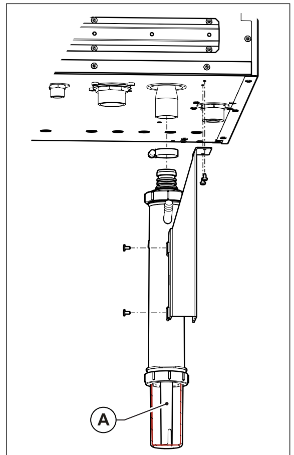
Рис. 10 Закріплення збірника
