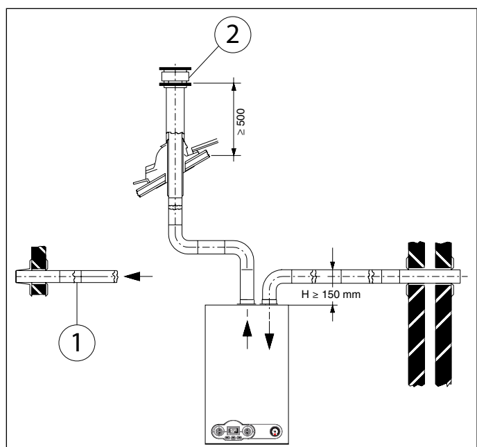
Рис. 10 Приклади системи збору повітря/викиду продуктів згоряння
