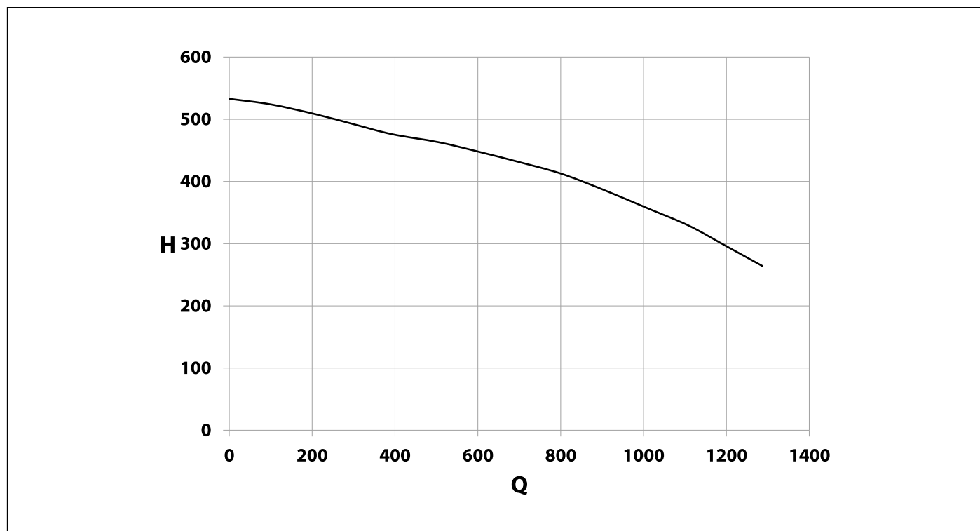
Рис. 15 Наявний напір
