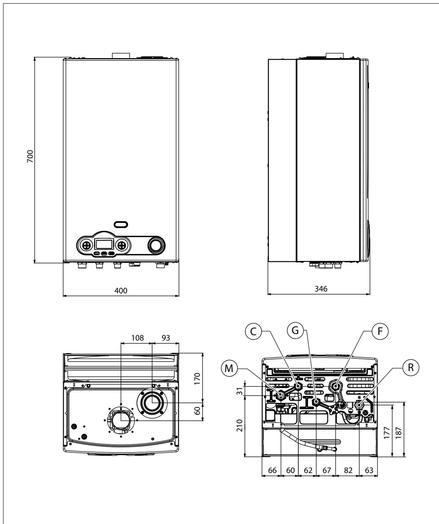
Рис. 3 Габарити
