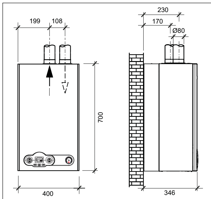
Рис. 9 Розміри для приєднання роздільних труб
