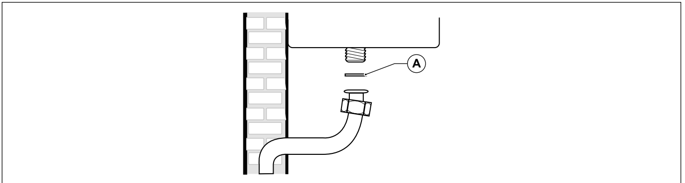
Рис. 13 Підключення газу
