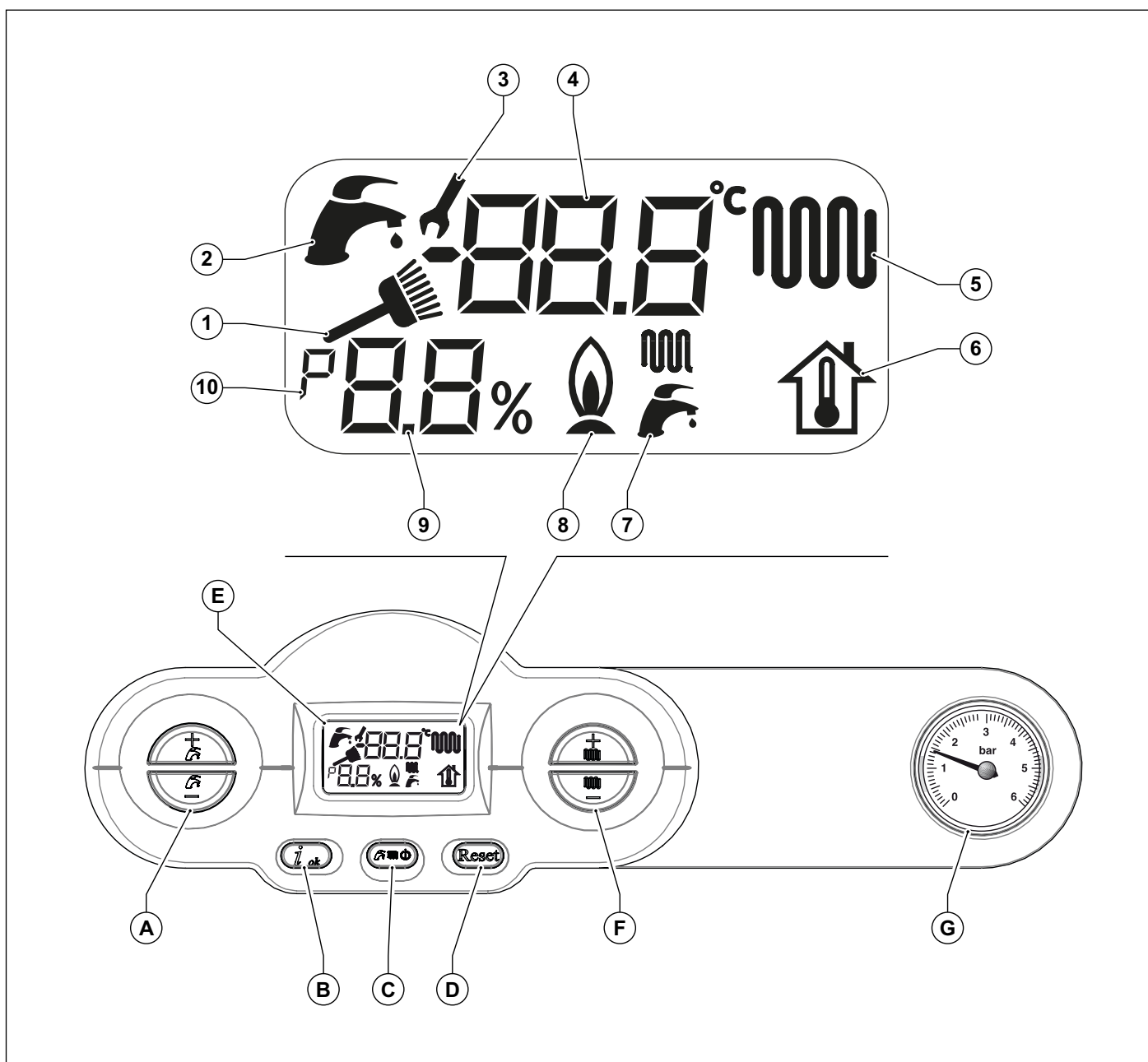
Рис. 1 Панель керування
