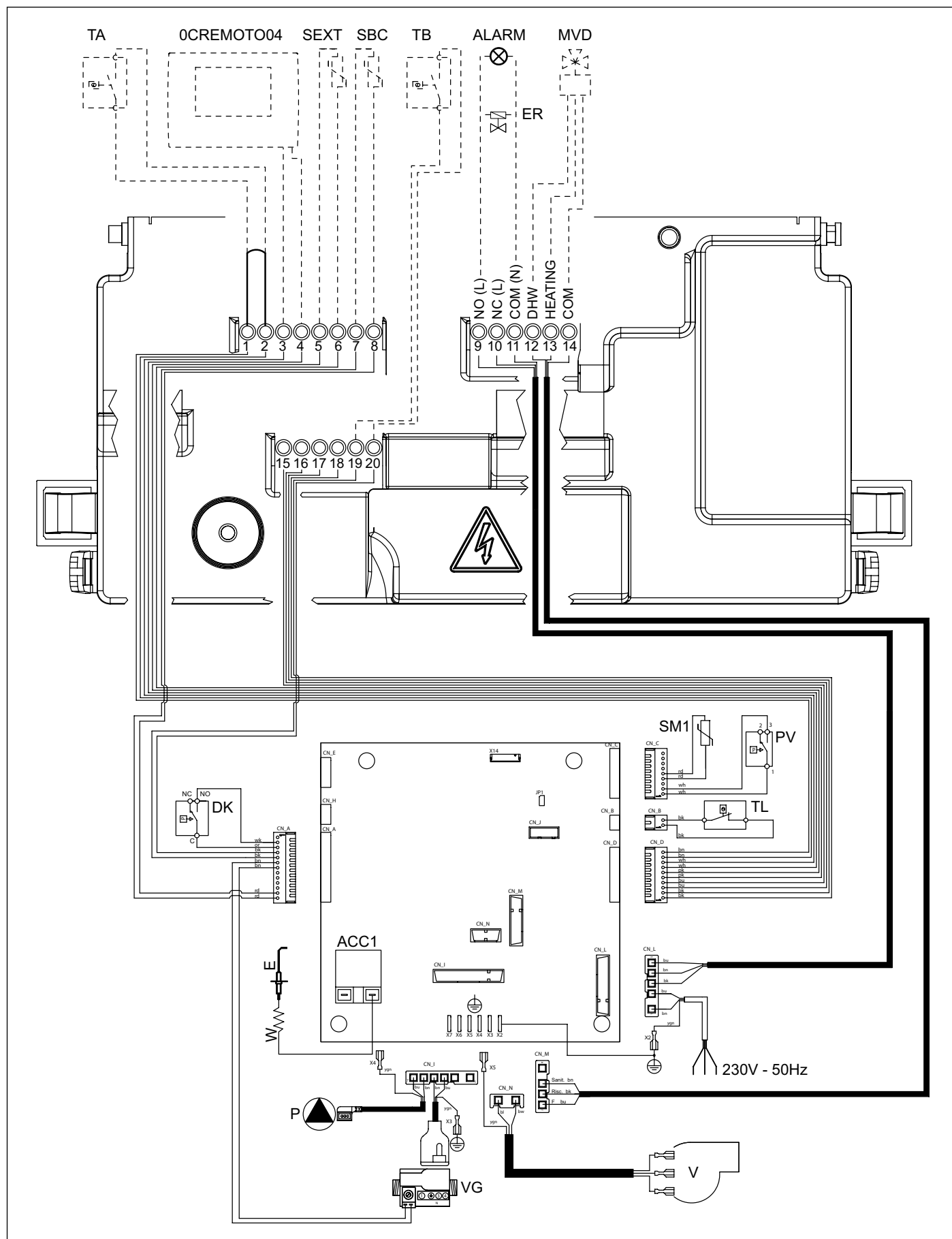
Рис. 18 Електрична схема RTFS
