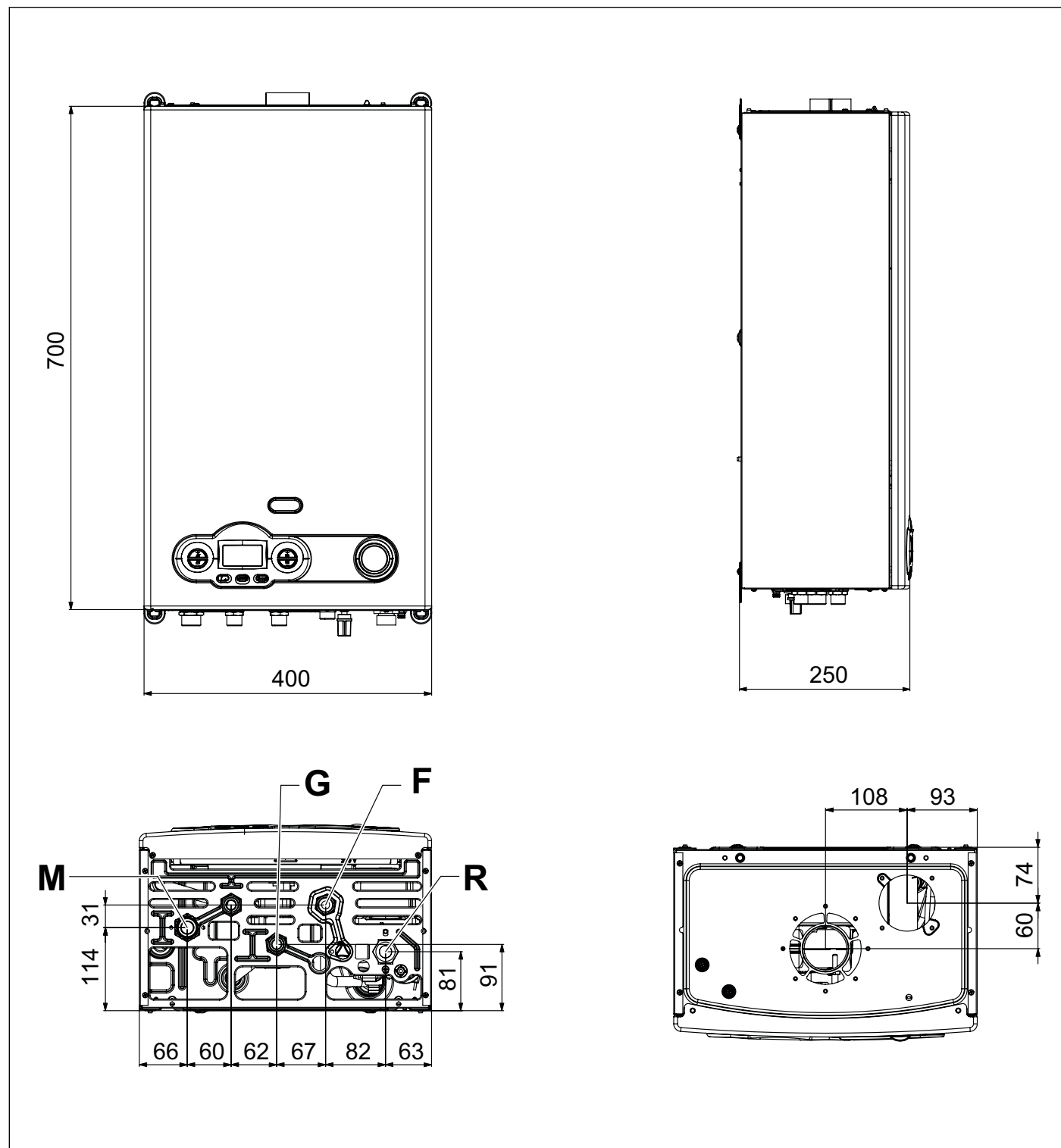
Рис. 3 Габарити RTFS
