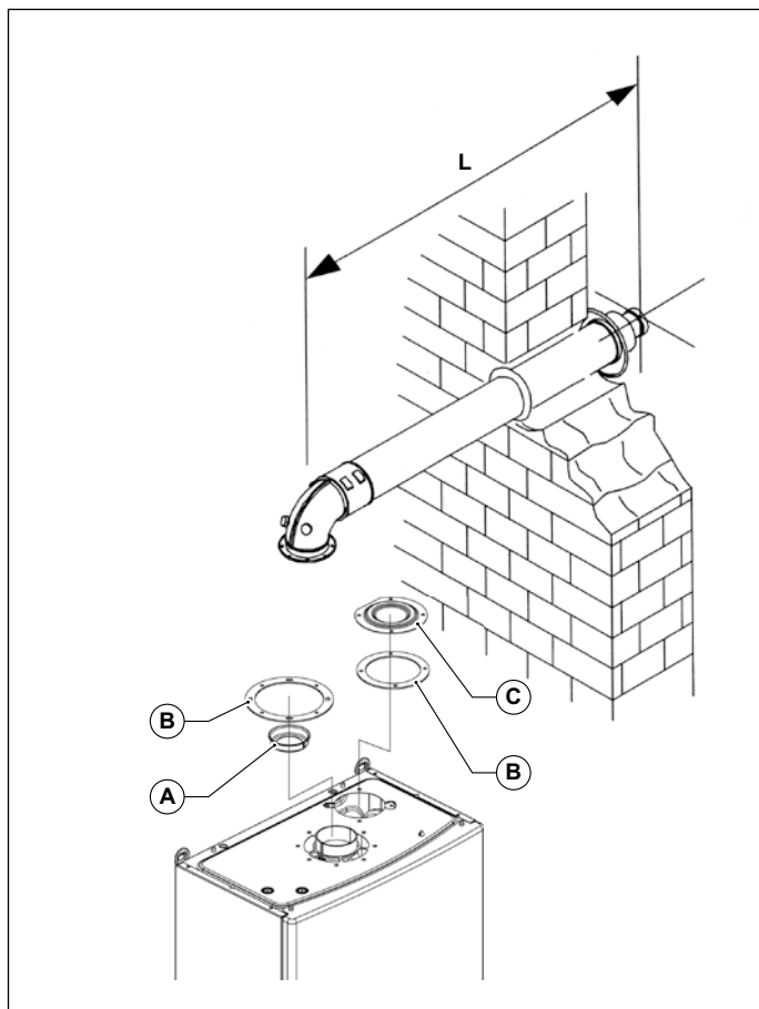
Рис. 8 0KITCONC00 (100/60 мм)
