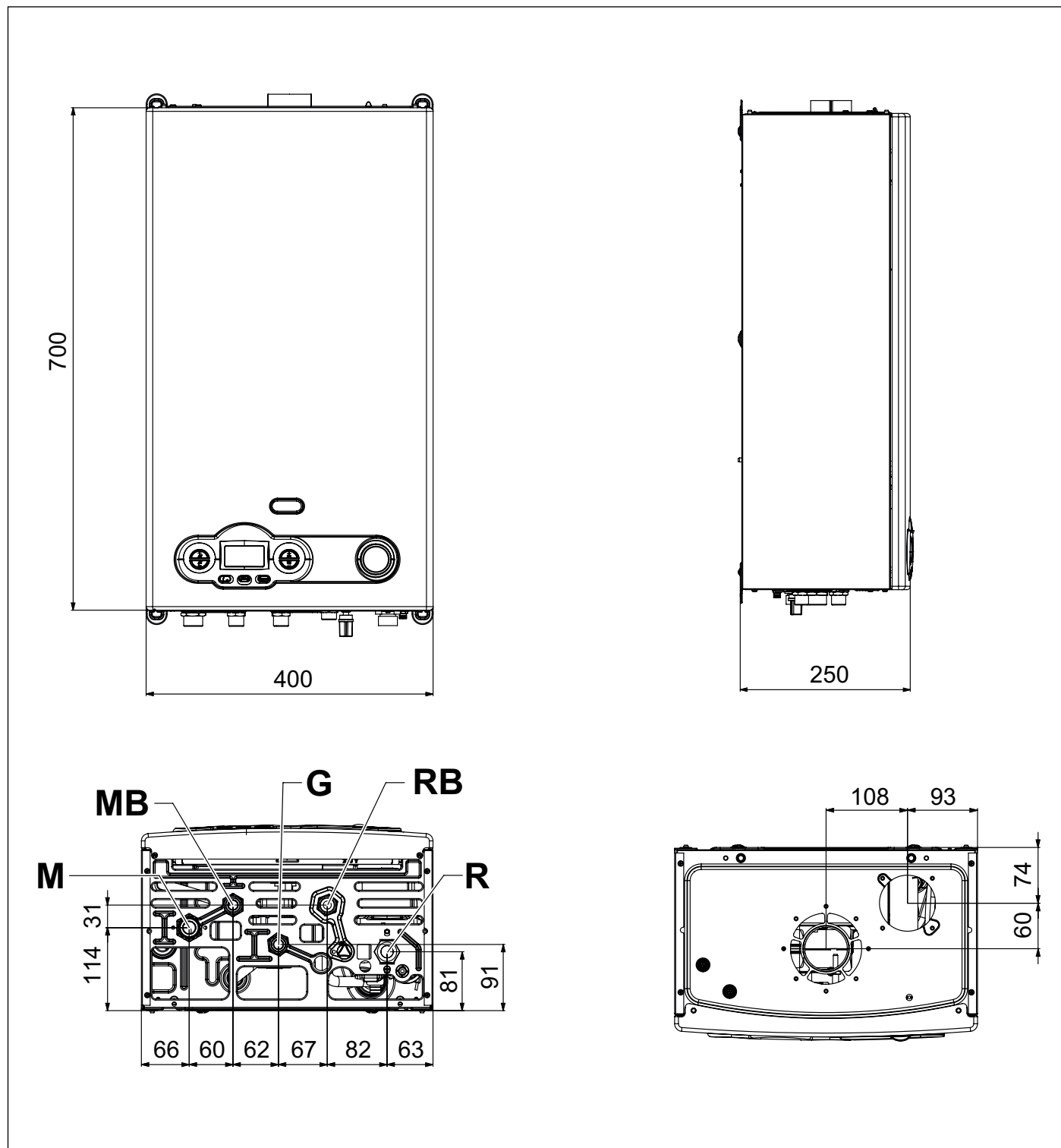
Рис. 4 Габарити RBTF5
