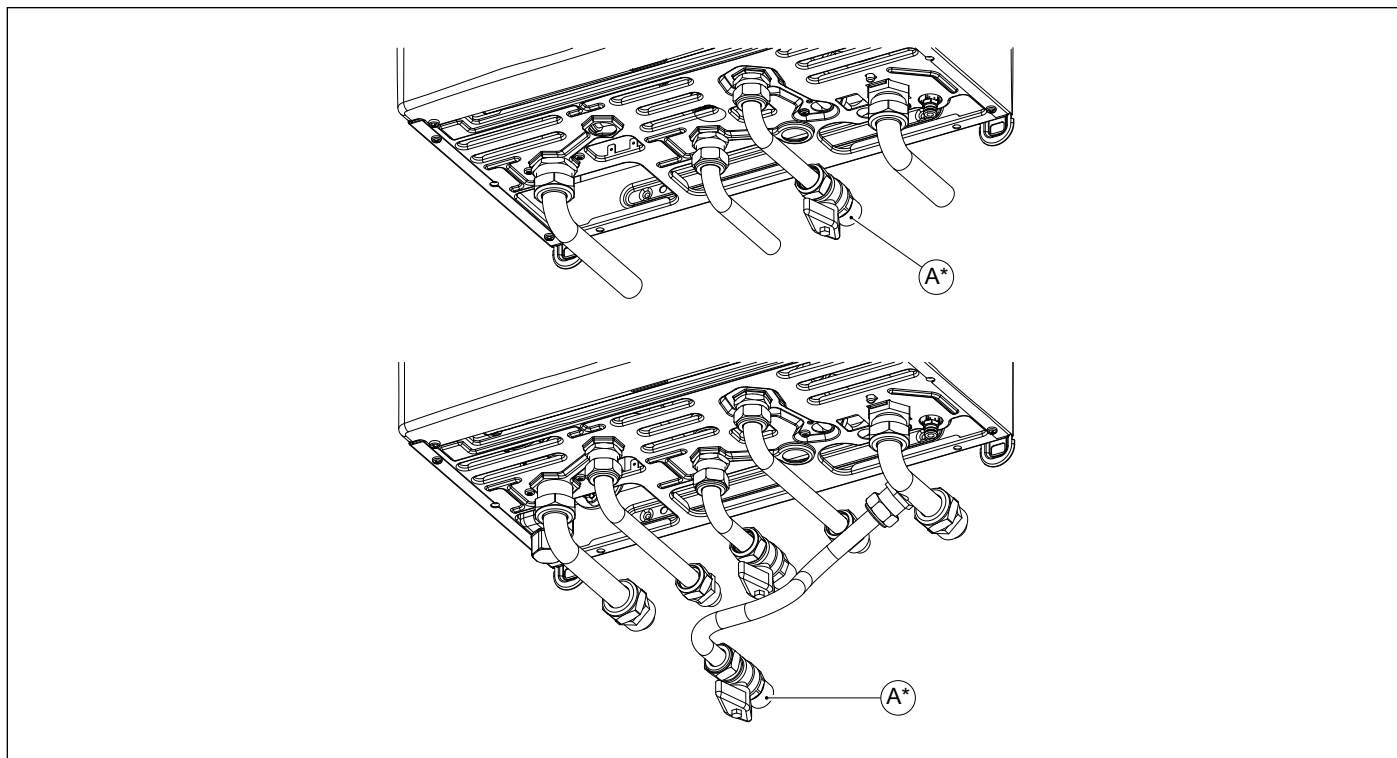
Рис. 2 Кран підживлення
