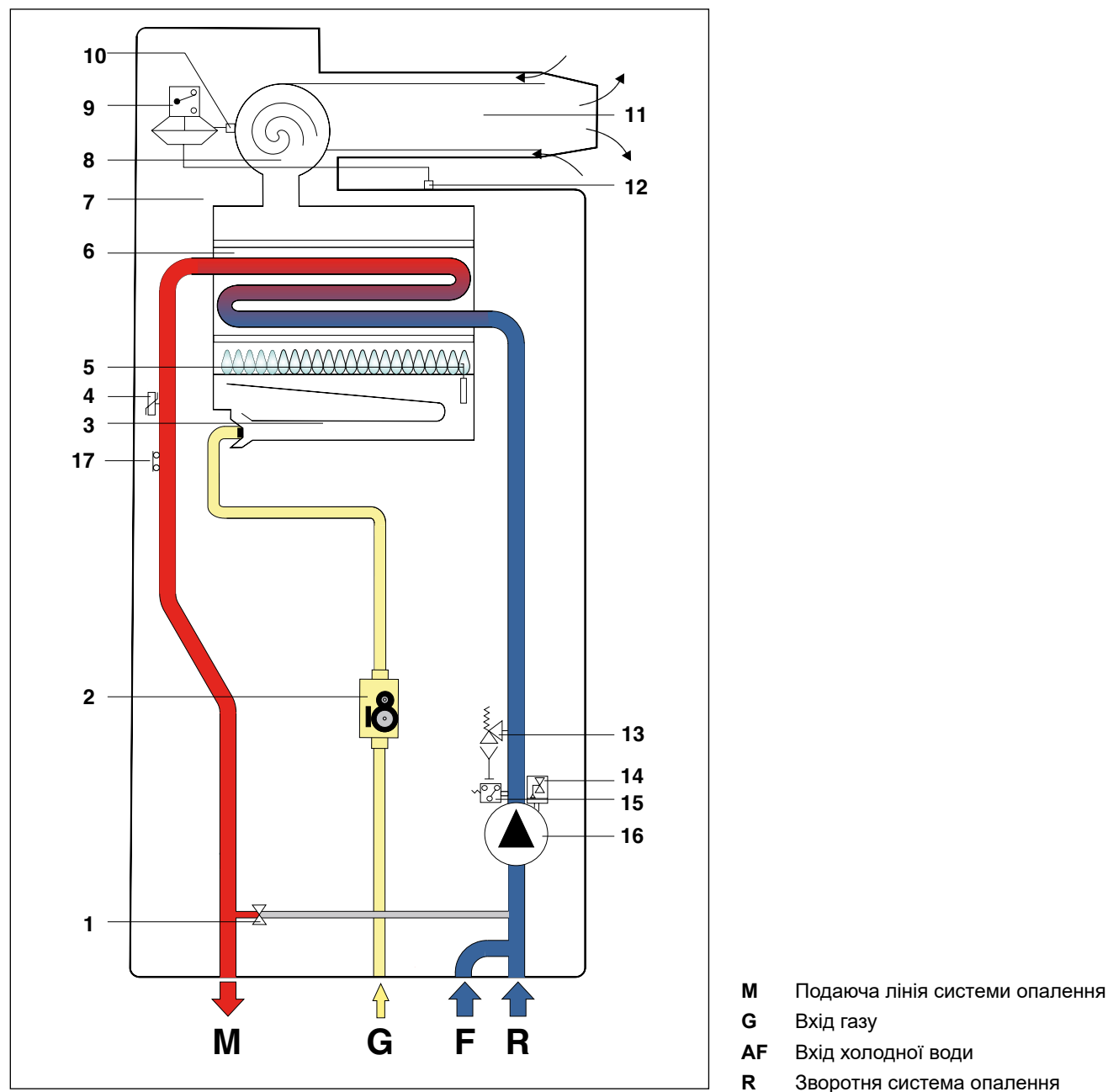
Рис. 5 Гідравлічна схема RTFS
