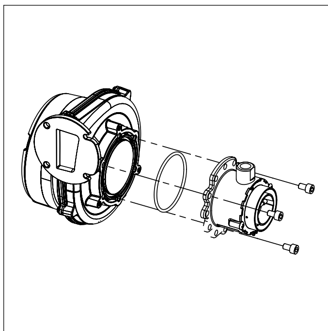
Fig. 42 Mezclador
