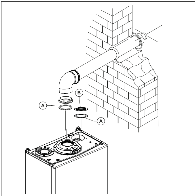
Fig. 14 Conductos coaxiales tipo C13 - C33
