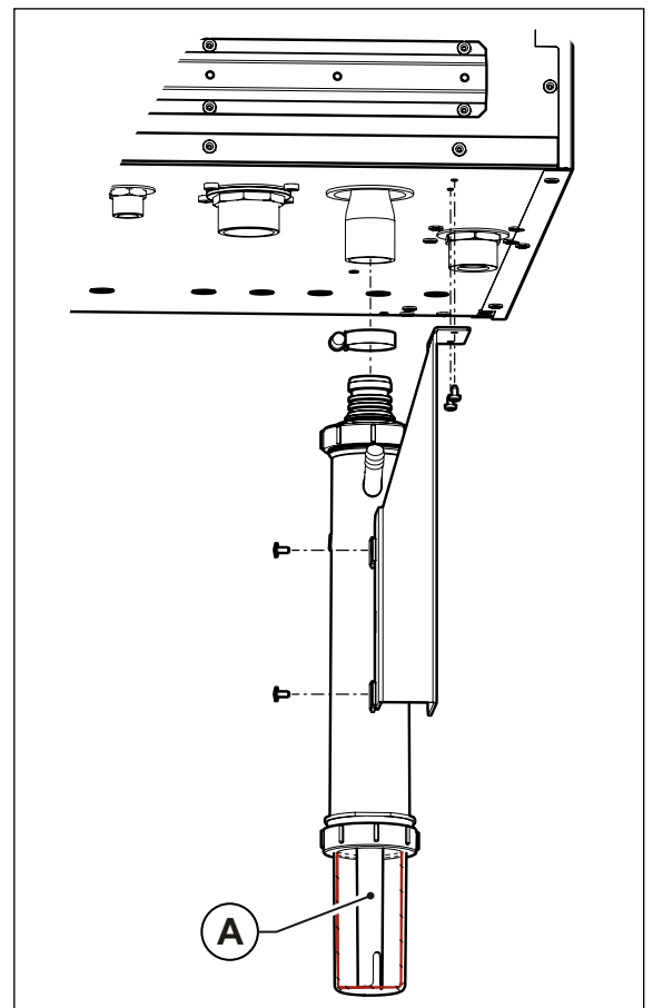
Fig. 10 Fijación del sifón
