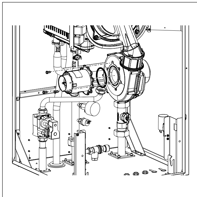
Fig. 33 Mezclador
