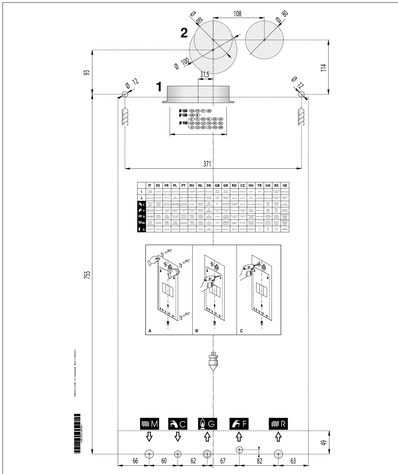
Рис. 11 Паперовий шаблон.
