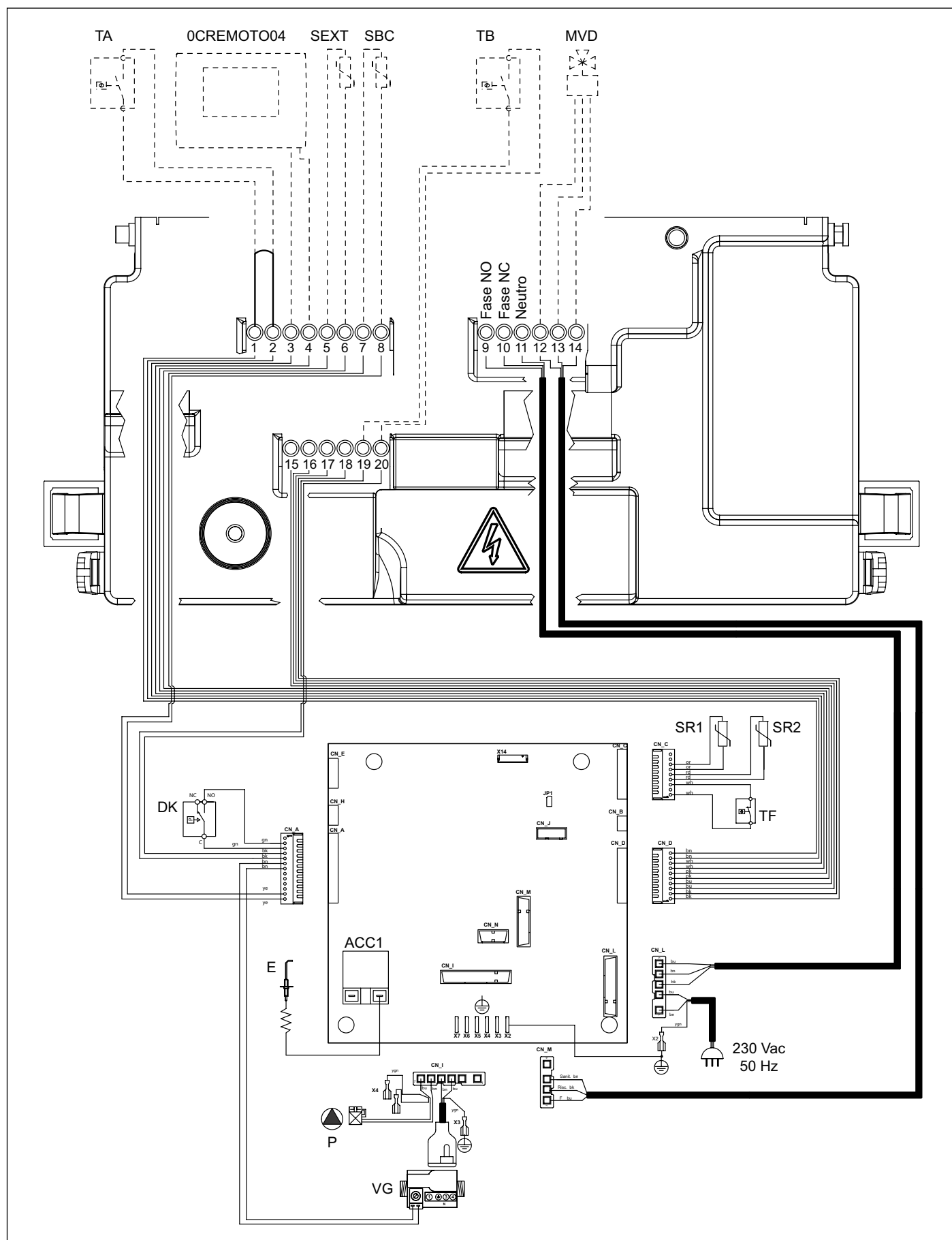
Рис. 28 Електрична схема RTN
