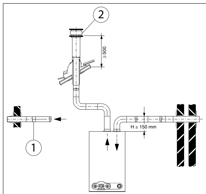
Рис. 18 Приклади системи забору повітря/викиду продуктів згоряння
