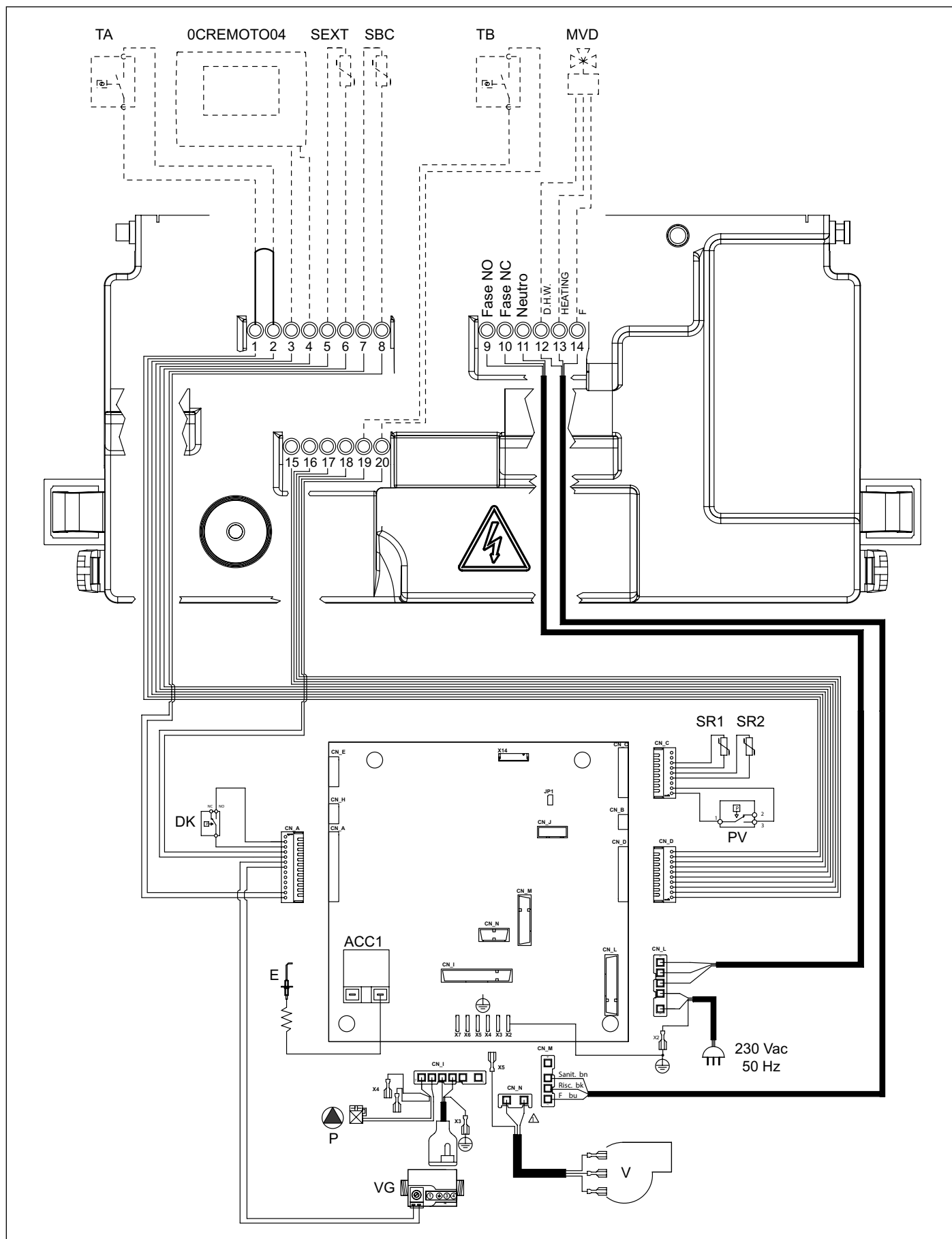
Рис. 25 Електрична схема RTFS
