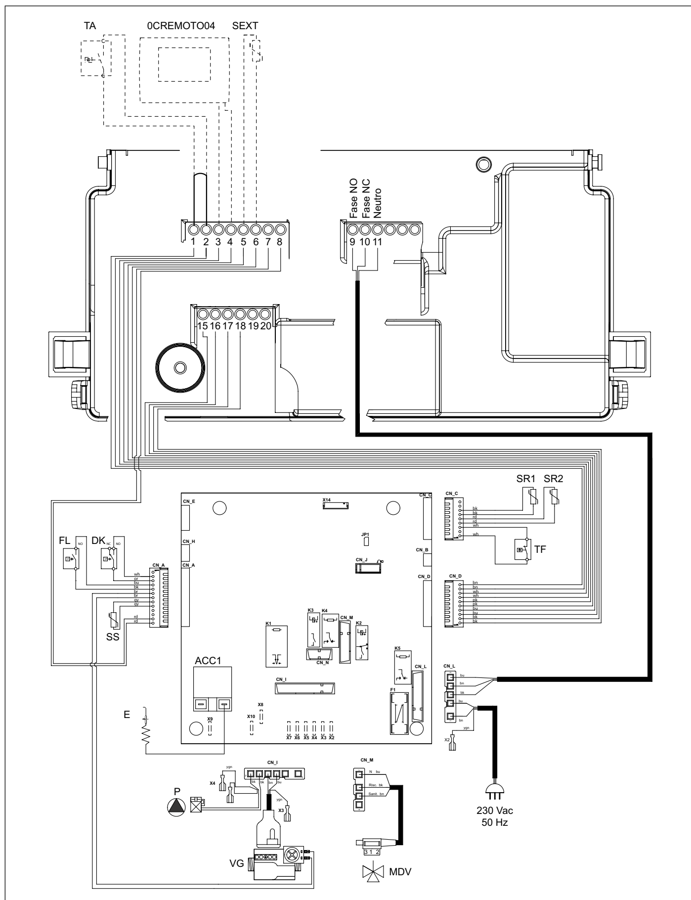
Рис. 27 Електрична схема CTN
