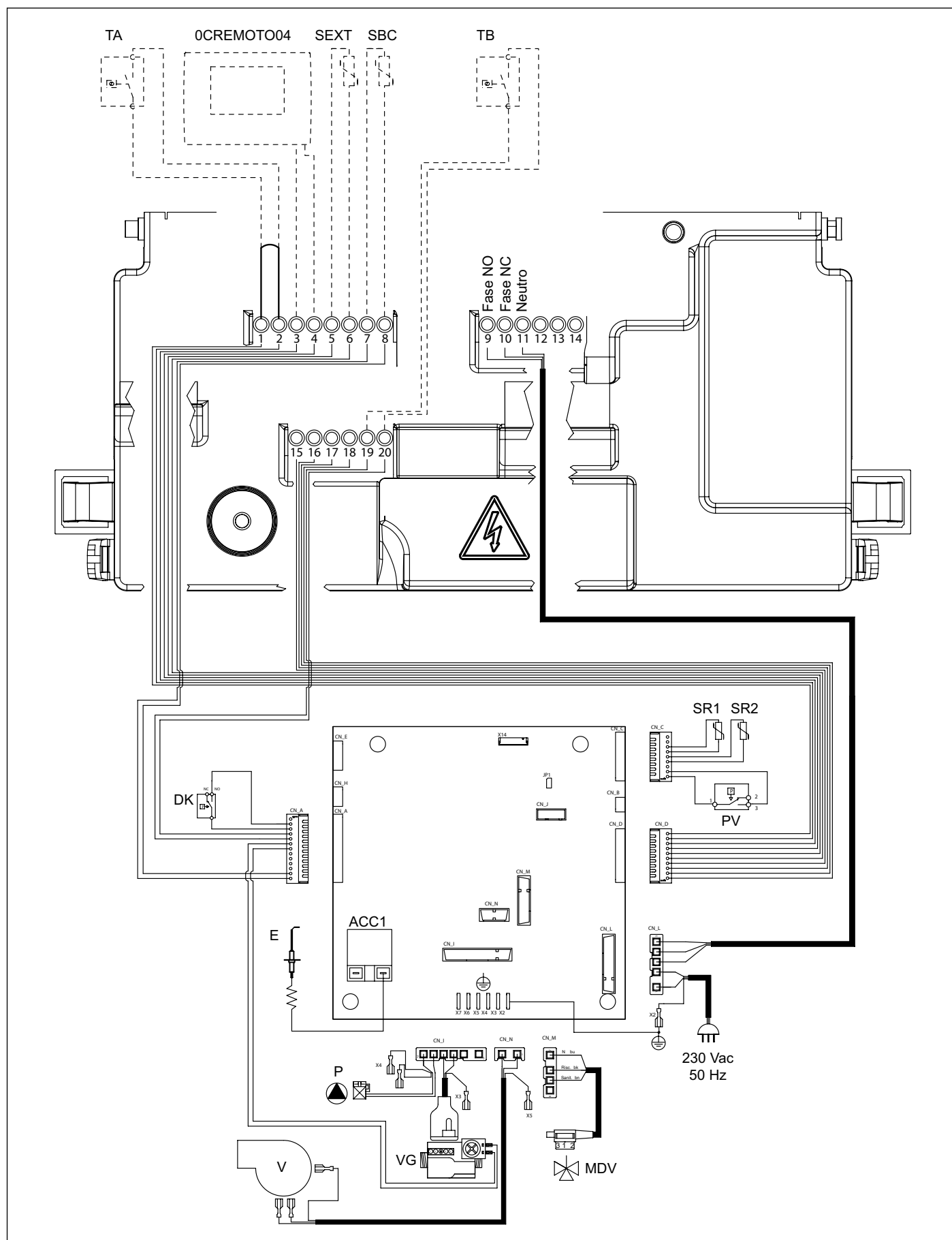
Рис. 26 Електрична схема RBTF5
