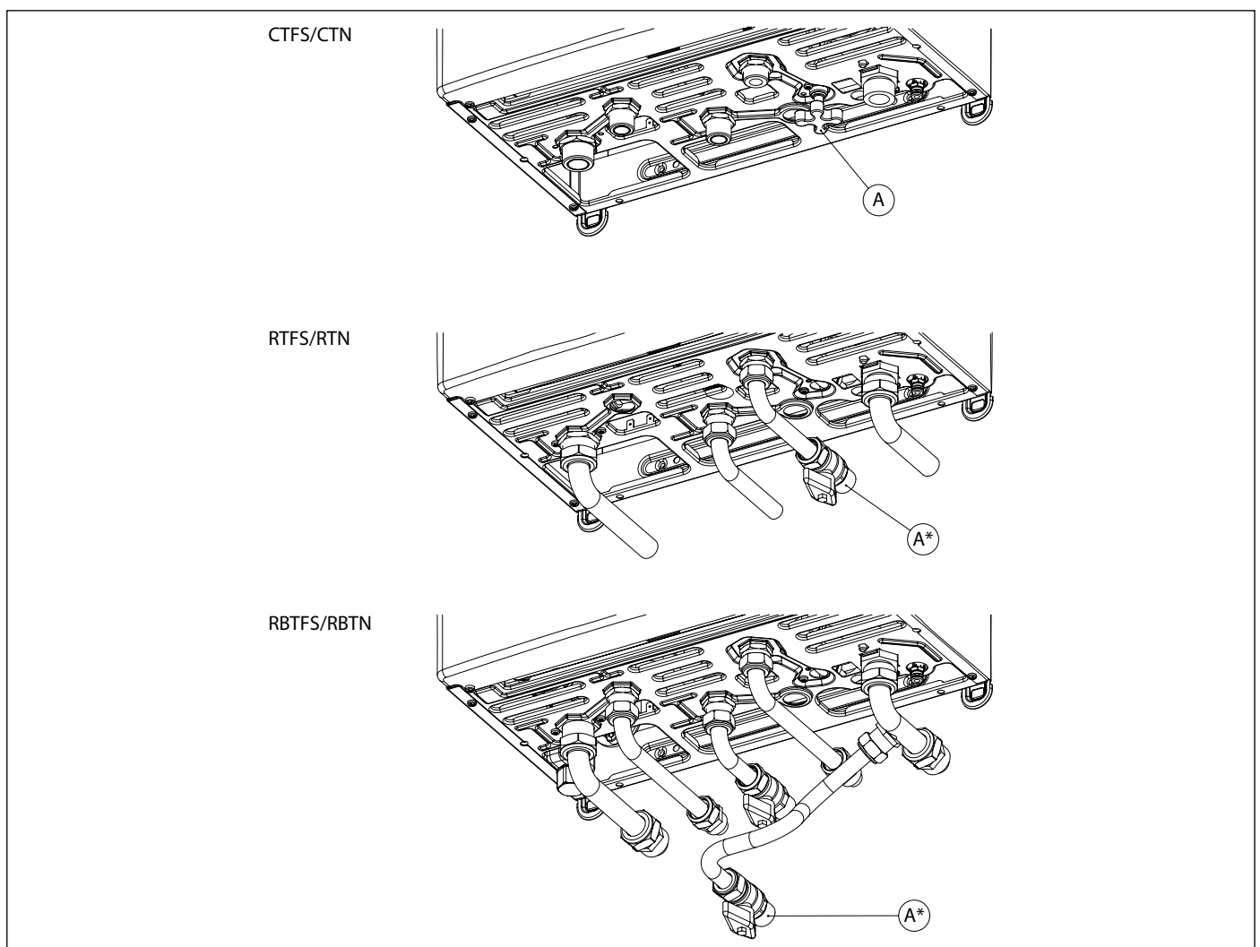
Рис. 2 Кран підживлення
