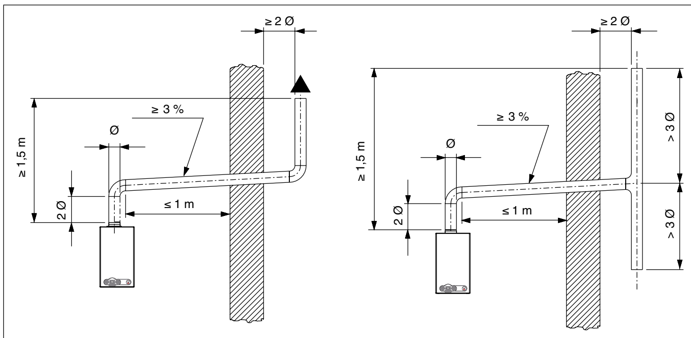
Рис. 6 Підключення димоходу до котла з відкритою камерою згоряння
