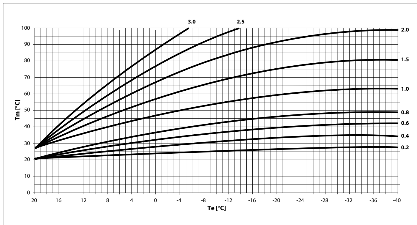
Рис. 24 Температурні криві
