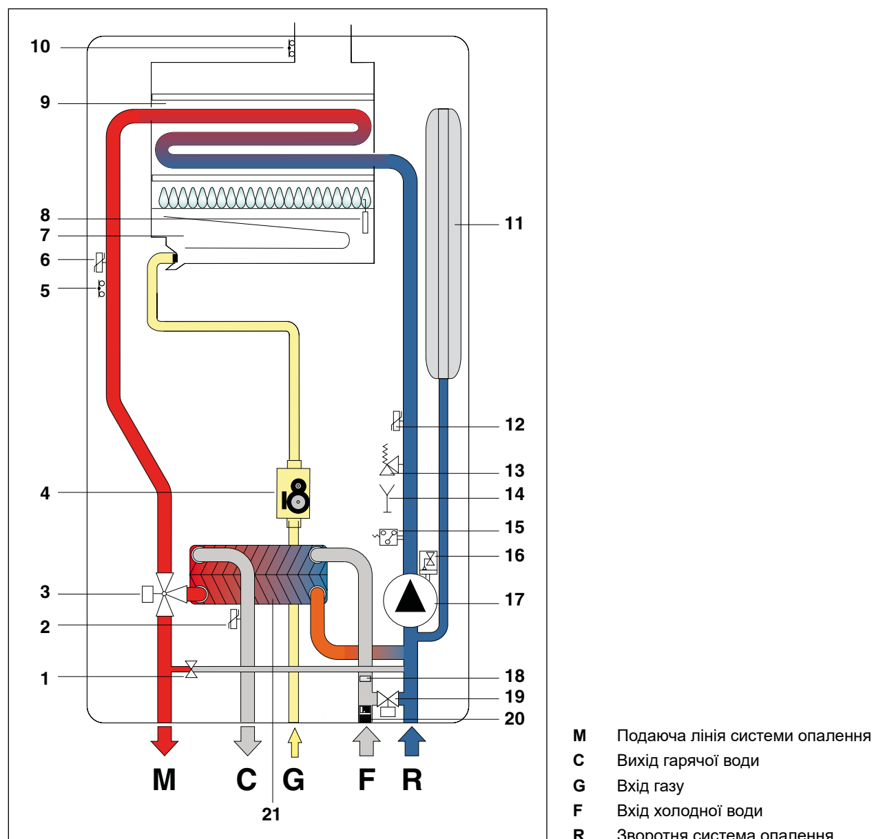
Рис. 4 Схеми гідравлічних підключень CTN
