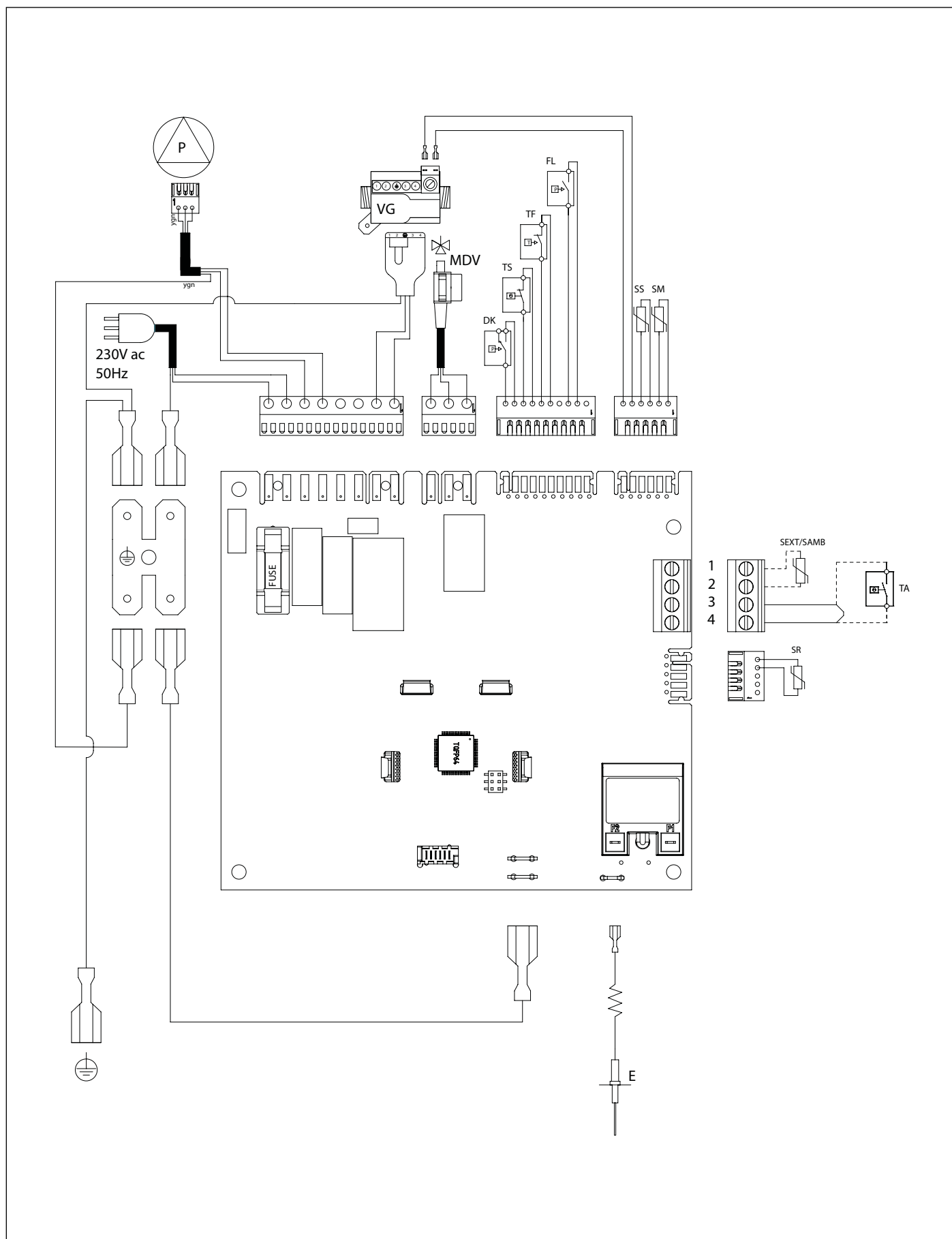
Рис. 11 Електрична схема СТН
